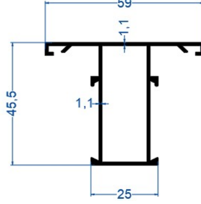
Aldoks Dar Orta Kayıt Profili
