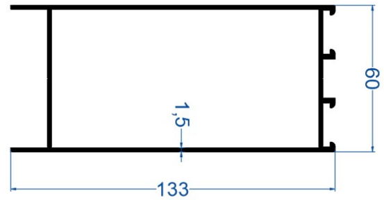
C-60 Etek Profili
