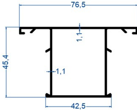
Aldoks Geniş Orta Kayıt Profili
