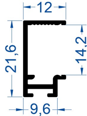
14 mm Fitilli Cam Contası
