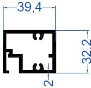
Alt & Üst Yatay Kayıt Profili
