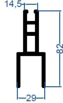
Isıcam Düz Kanat
