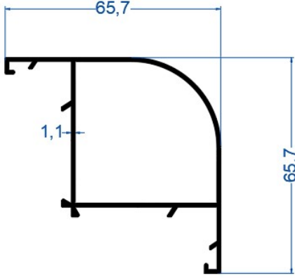
Aldoks Köşe Profili
