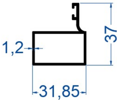
Yan Dikme Profili
