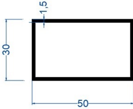
30*50*1,5 mm Kutu Profil
