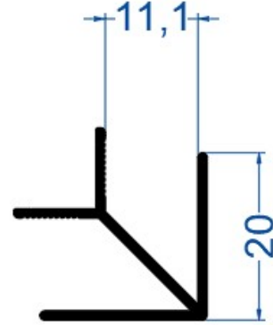
19Y04 Köşe Çavuşu
