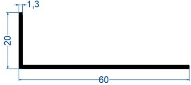
20*60*1,3 mm Düz Köşebent
