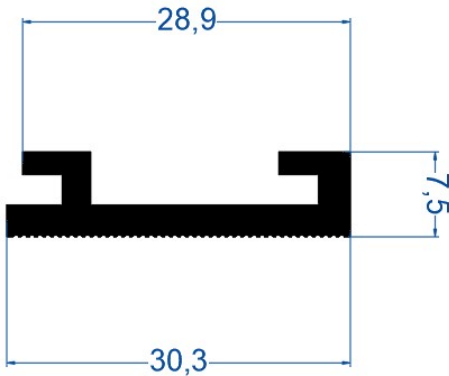
ERG AS 02 Askı Üst Profil
