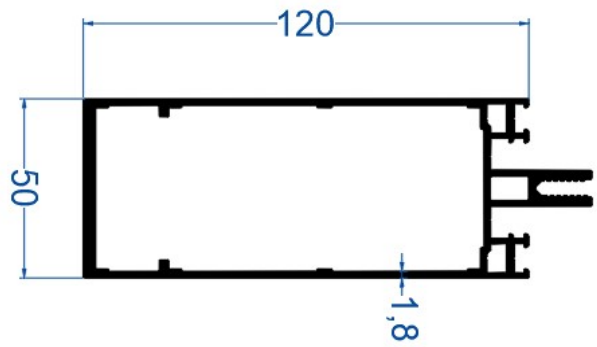
120'lik Düşey Cephe Profili
