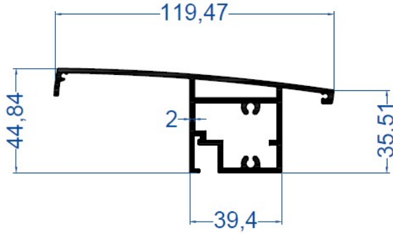
Haraketli Yatay Kayıt Profili
