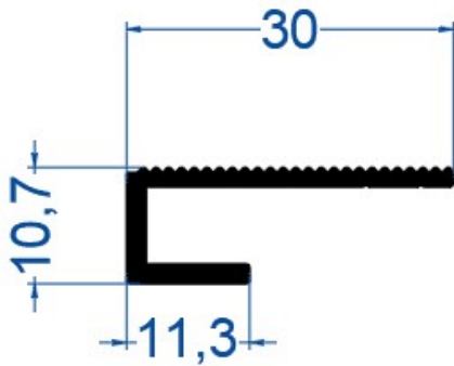
Sinter Orta Profil
