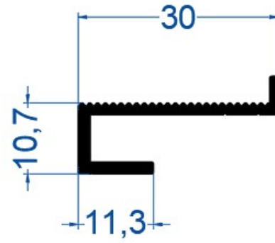
Sinter Alt Profil
