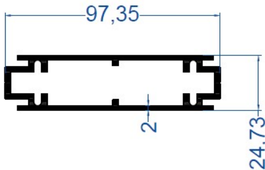
Adaptör Kasa Profili
