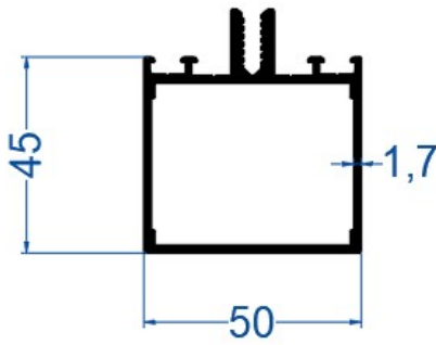
45'lik Yatay Cephe Profili
