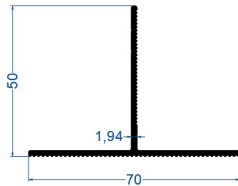
50*70*1,9 mm "T" Profil
