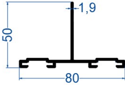
80*50*1,9 Çift Klipsli T Profili
