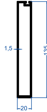
20X135 1,5MM KUTU FİTİLLİ
