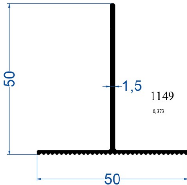
50*50*1,5 mm "T" Profil
