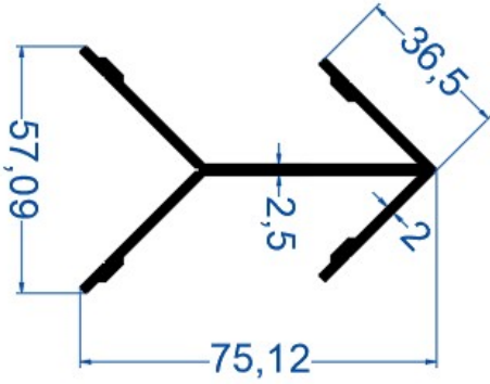
C-60 Çavuş Profili
