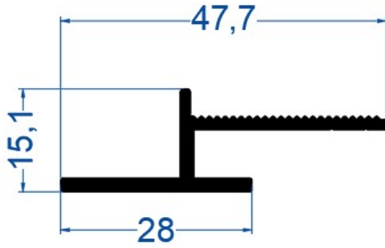
Sinter Üst Profil
