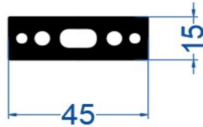
Ana Dikey Kayıt Profili
