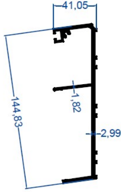
Duvar Bağlantı & E Kasa Profili
