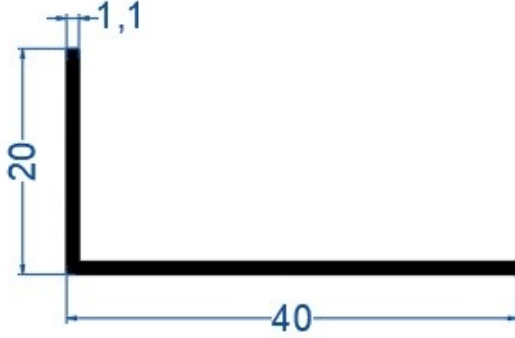
20*40*1,1 mm Düz Köşebent
