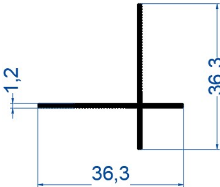
19Y06 Köşe Profili
