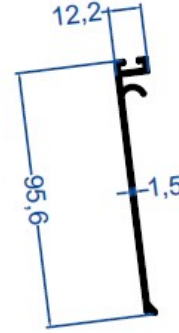
Figürlü Dere Kapak Profili
