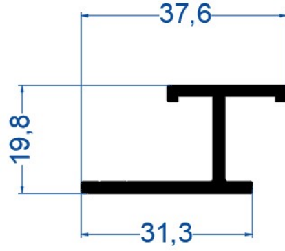
Sinter Klips Profil Yarım
