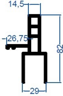
Isıcam Fitilli & Kenetli Kanat
