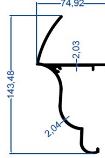
Figürlü Dere Kapak Profili
