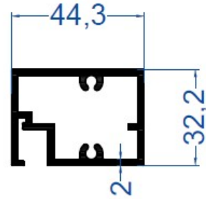
Sabit Alt & Üst Yatay Kayıt Profili
