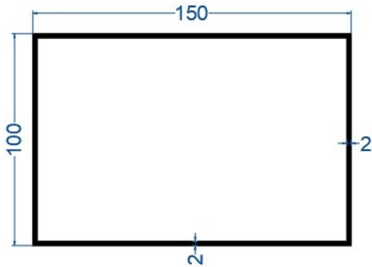
100*150*2,0 mm Kutu Profil
