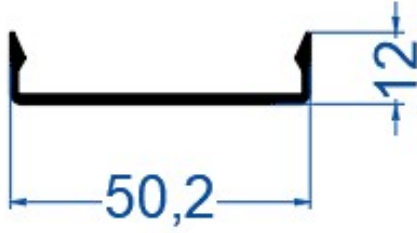
12 mm Kapak Profili
