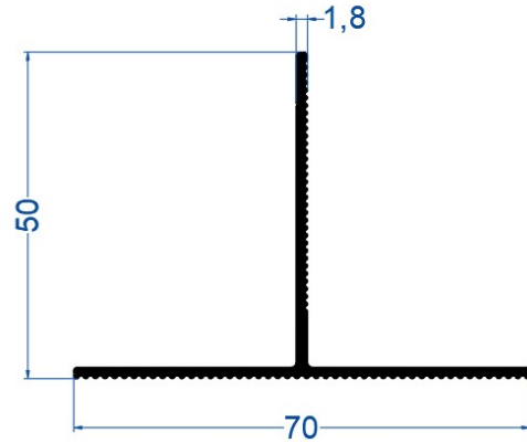
50*70*1,8 mm "T" Profil
