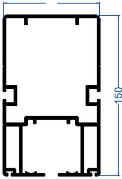
ANA RAY PROFİLİ 90'LIK EKO - TIRTIKSIZ
