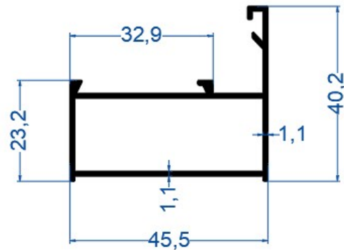
Aldoks Dar Kasa Profili
