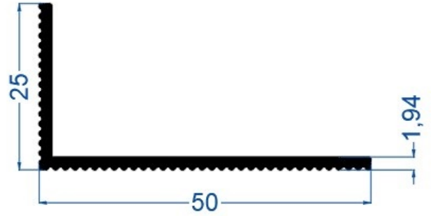
25*50*1,9 mm Tırtıklı "L" Profil E-1281 0,350 m/kg
