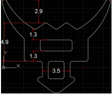
DÜZ ROLİNG VE BİOCLİMATİC PANEL FİTLİ ERG-06
