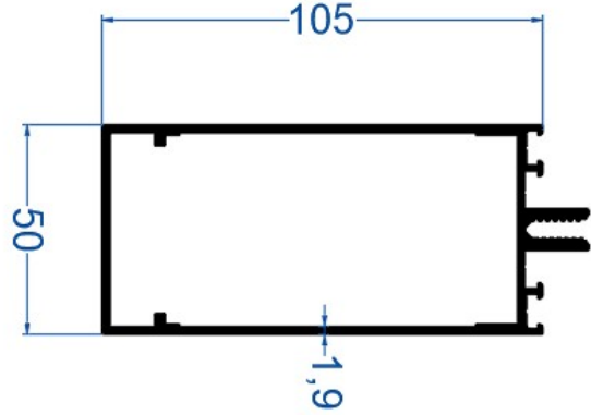
105'lik Yatay Cephe Profili
