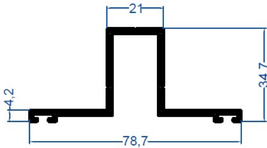
Isıcam Orta Kayıt Profili
