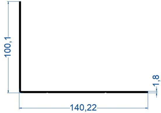
100*140*1,8 mm Düz Köşebent
