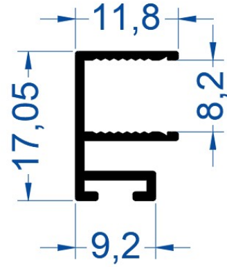
8 mm Fitilli Cam Contası
