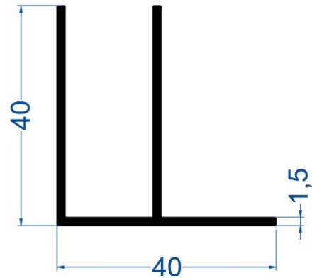
"F" Profil 16 mm
