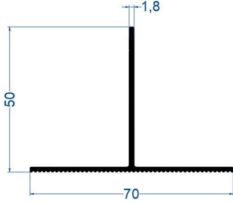
50*70*1,8 mm "T" Profil
