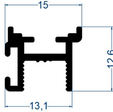
10 mm Kanat Profili
