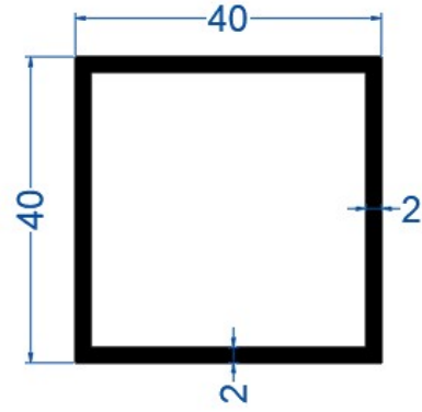
40*40*2,0 mm Kutu Profil
