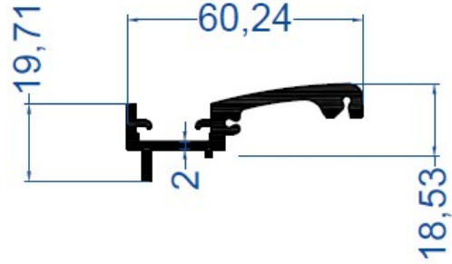
Adaptör Yan Kapak Profili
