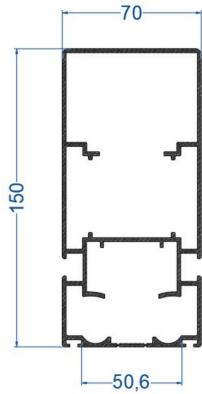
Ana Ray Profili 70'lik - Desteksiz
