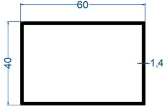
40*60*1,4 mm Kutu Profil
