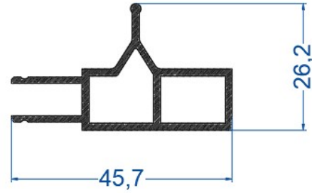
Profil Adı E-1952 0,520 m/kg
