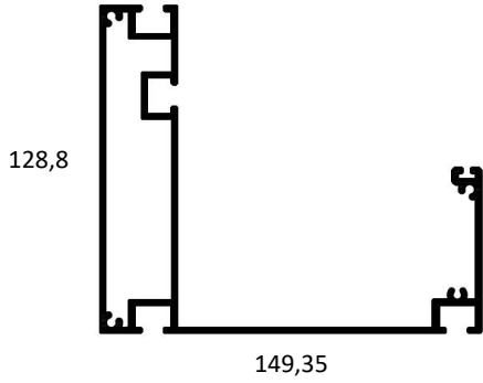
Pergola Dere Profili
