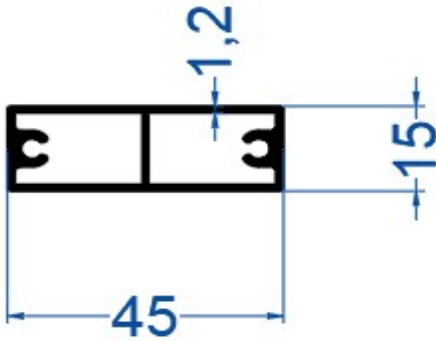
Dikey Ara Kayıt Profili
