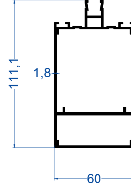
Orta Kayıt Profili
