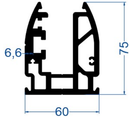
75 mm Baza Profili
