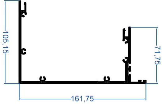
Kutu Dış Profili
