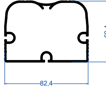
BÜYÜK ARMUT PROFİLİ
