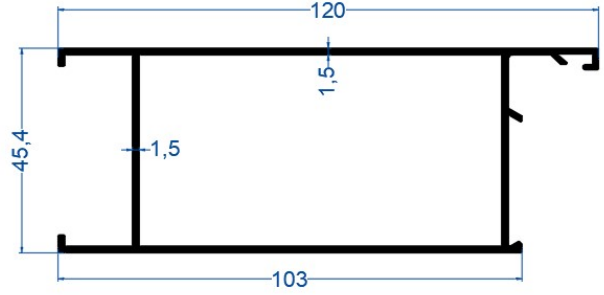
Aldoks Isıcam Çıta
