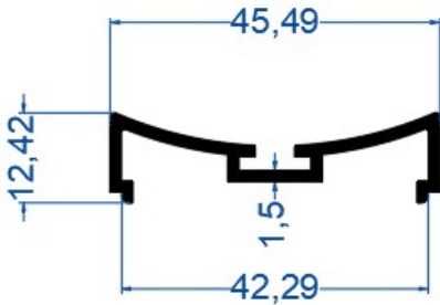
Aldoks Çarpma Kapı Adaptörü
