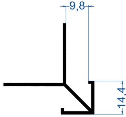
19Y03 Köşe Çavuşu
