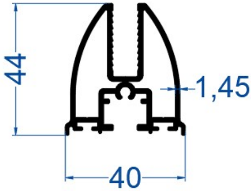
"Fırtına" Kanat Profili
