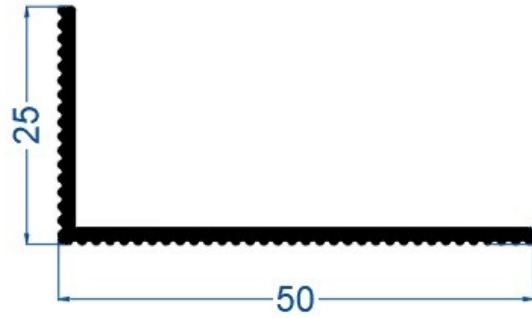
25*50*1,8 mm Tırtıklı "L" Profil E-1282 0,315 m/kg
