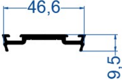
Alt Baskı Profili
