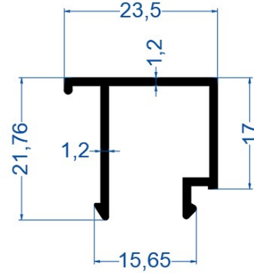
C-60 Tek Cam Çıtası
