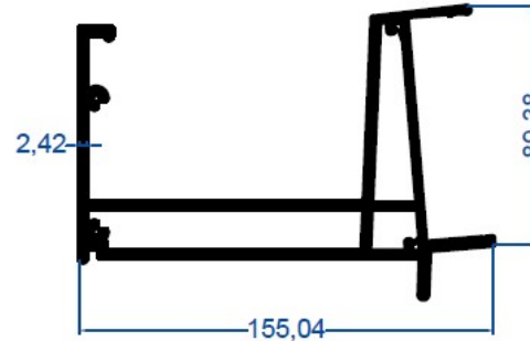
Veranda Destekli Dere Profili
