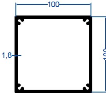
Yan & Köşe Kayıt Profili
