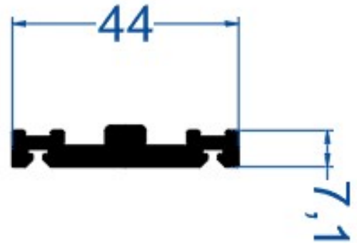
75 mm Baza Sıkıştırma Profili
