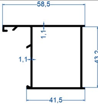
Aldoks Geniş Kasa Profili
