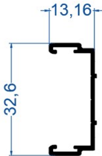
Profil Adı E-1923 0,179 m/kg
