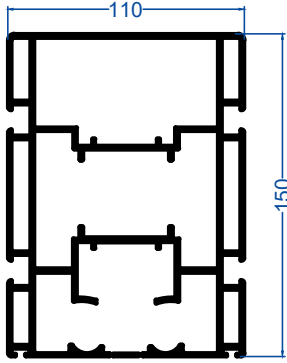
ANA RAY PROFİLİ 110'LUK - TIRTIKSIZ
