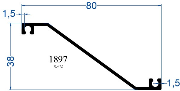
Zikov Askı Profili
