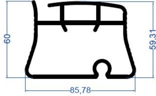
Patlatmalı Büyük Armut Profili
