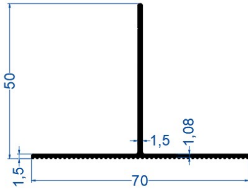
50*70*1,5 mm "T" Profil
