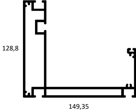
Pergola Dere Profili
