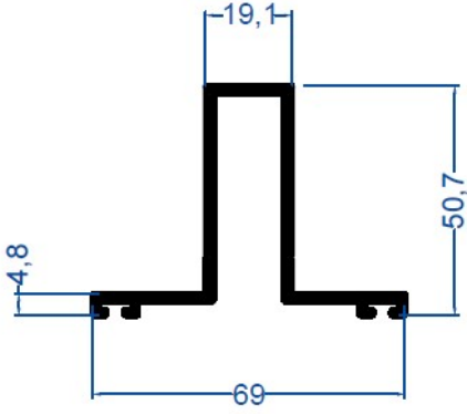
Tek Cam Orta Kayıt Profili
