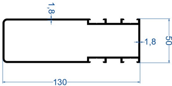
C-60 Takviye Kasa Profili
