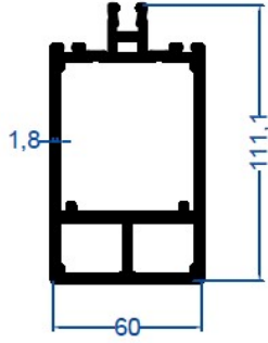
Destekli Orta Kayıt Profili
