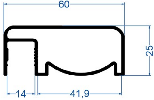
Kare Yan Kanallı Üst Baza
