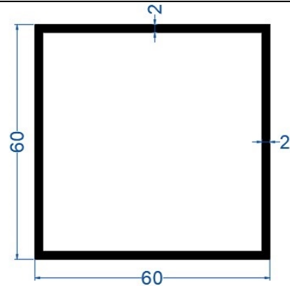
60*60*2,0 mm Kutu Profil
