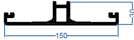
Alt Kasa Profili
