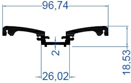
Adaptör Orta Kapak Profili
