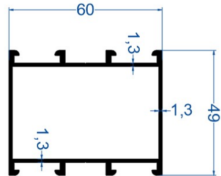
C-60 Etek Profili
