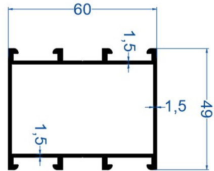
C-60 Kasa Profili 1,50 mm
