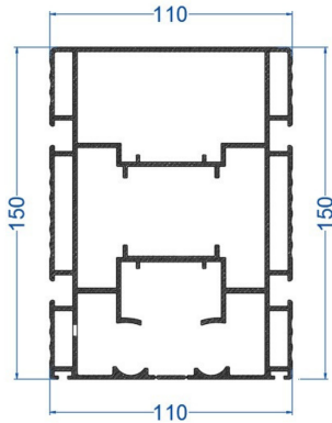
Ana Ray Profili 110'luk - Tırtıklı
