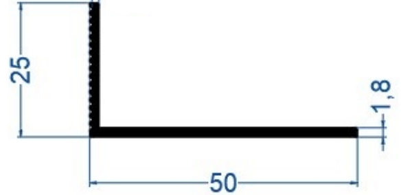
25*50*1,8 mm Tırtıklı Kısa Kenar E-1880 0,328 m/kg
