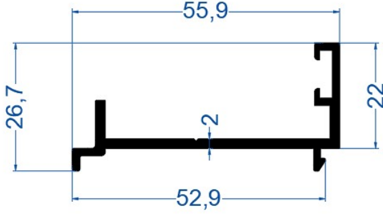
C-60 Adaptör Profili
