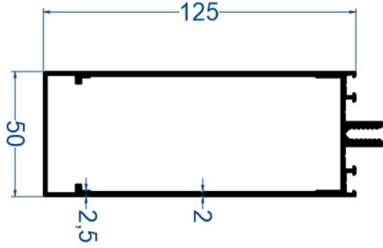
125'lik Yatay Cephe Profili
