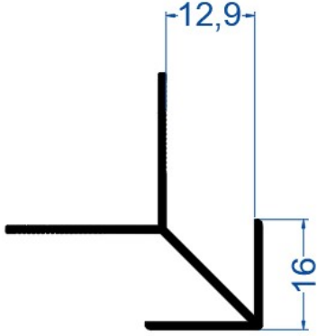
19Y01 Köşe Çavuşu
