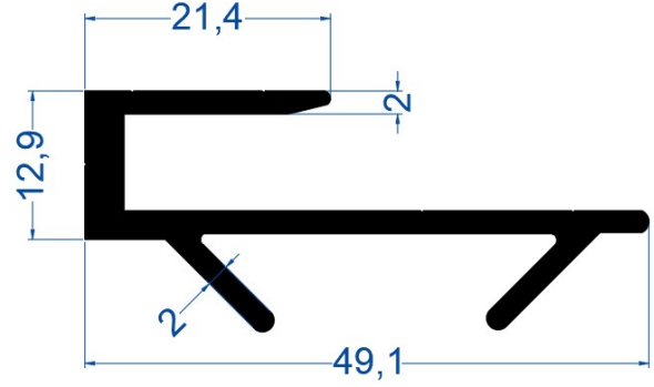
Zikov Askı Profili
