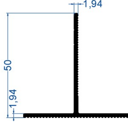
50*50*1,9 mm "T" Profil
