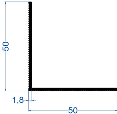
50*50*1,8 mm Köşebent E-1029 0,440 m/kg
