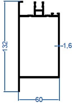
Yan & Köşe Kayıt Profili
