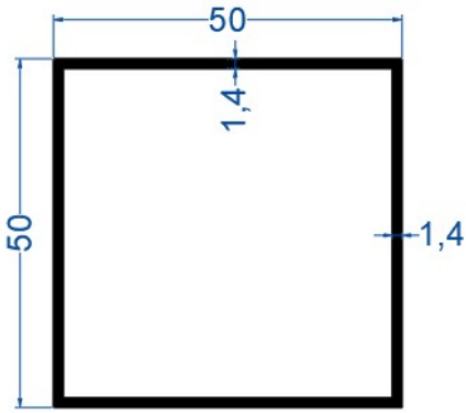
50*50*1,4 mm Kutu Profil
