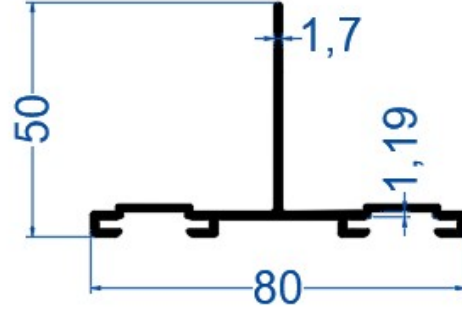
80*50*1,7 Çift Klipsli T Profili
