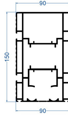
Ana Ray Profili 90'lık - Tırtıklı
