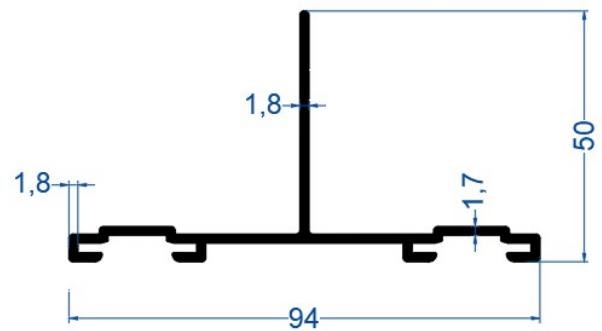
94*50*1,8 Çift Klipsli T Profili
