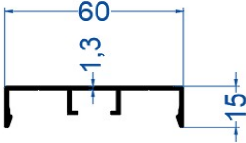
Üst Baza Profili
