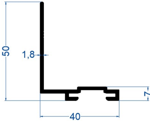
40*50*1,8 Klipsli L Profili
