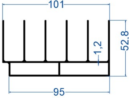
Eşikli Yan & Üst Kasa Profili
