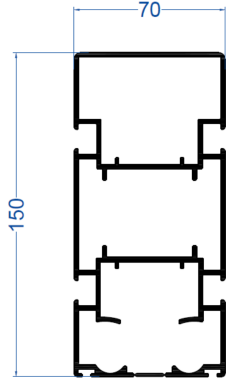
Ana Ray Profili 70'lik - Düz
