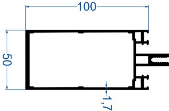
100'lük Düşey Cephe Profili
