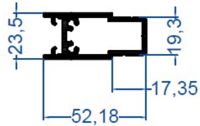
Ray Kapama Profili
