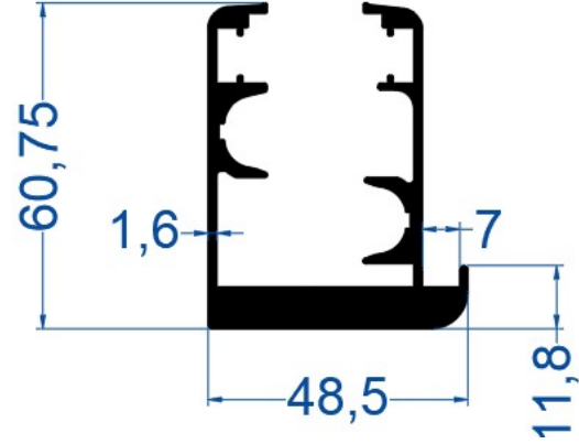
Damlalıklı Kasa Profili
