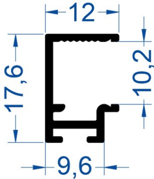
10 mm Fitilli Cam Contası
