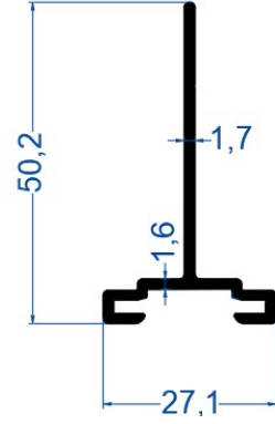
27*50*1,7 Tek Klipsli T Profili
