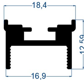
12 mm Kanat Profili
