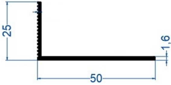
25*50*1,6 mm Tırtıklı Kısa Kenar E-2098 0,310 m/kg
