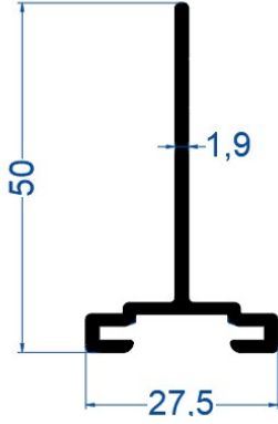
27*50*1,9 Tek Klipsli T Profili
