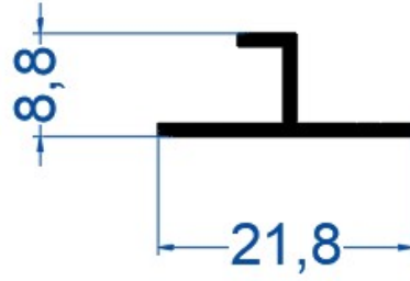
Derz Çıtası 8,8'lik
