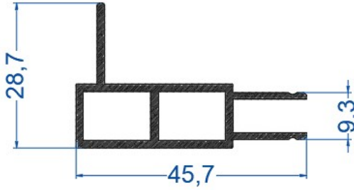
Profil Adı E-1917 0,534 m/kg
