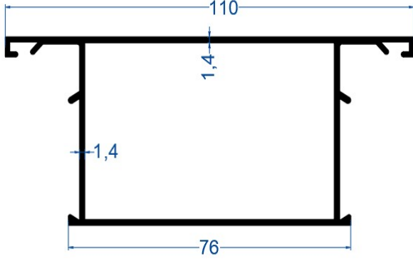
Aldoks Baza Orta Kayıt Profili
