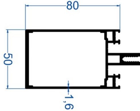
80'lik Düşey Cephe Profili
