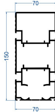
Ana Ray Profili 70'lik - Tırtıklı
