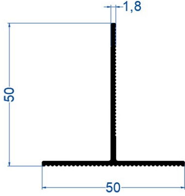
50*50*1,8 mm "T" Profil
