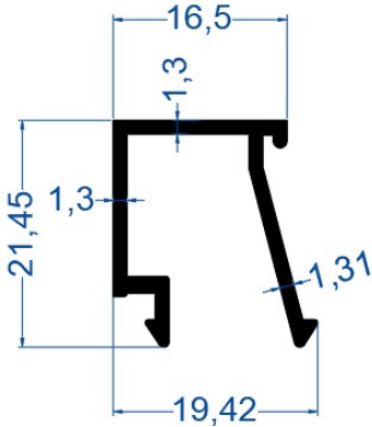
C-60 Isı Cam Çıtası
