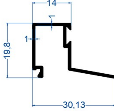
Aldoks Isıcam Çıta
