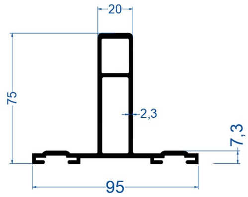
75*95*2,3 mm "T" Kutu Profil
