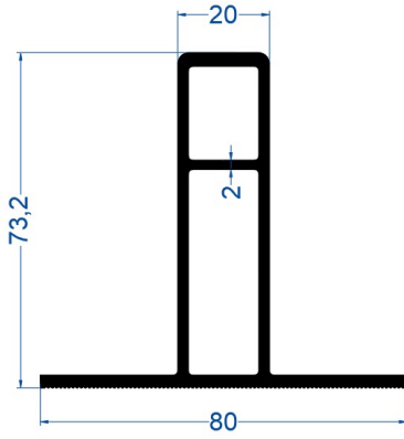
73*80*2,0 mm "T" Kutu Profil
