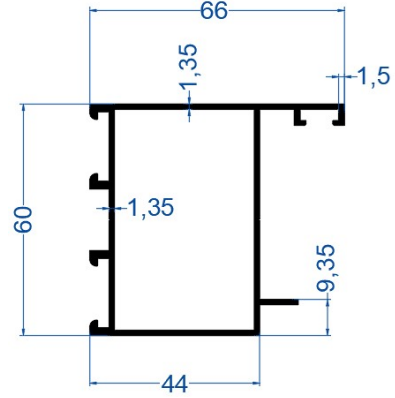
C-60 Kanat Profili
