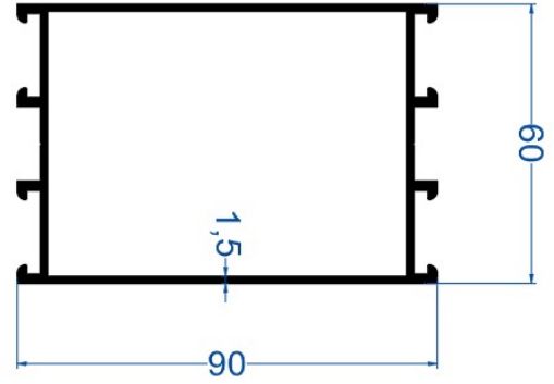
C-60 Geniş Kasa Profili
