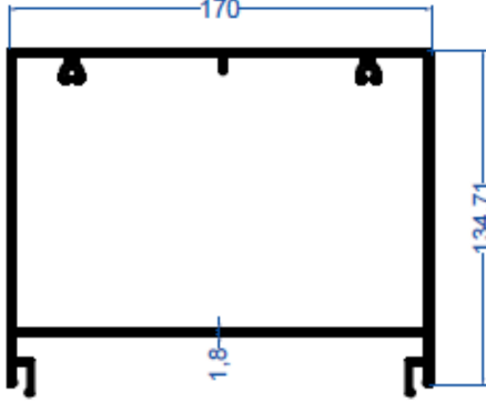
Taşıyıcı Kutu Profili
