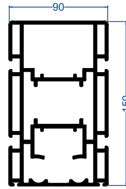
ANA RAY PROFİLİ 90'LIK - TIRTIKSIZ
