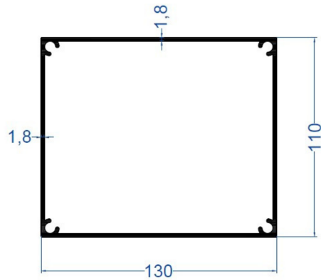
Kutu Profili 110X130
