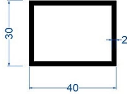
30*40*2,0 mm Kutu Profil
