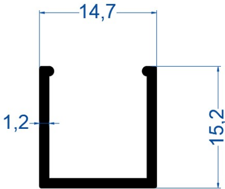
19Y05 "U" Profil
