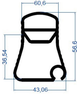
Patlatmalı Küçük Armut Profili
