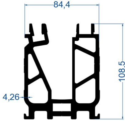
108,5 mm Baza Profili
