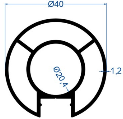
Yuvarlık Dikme 40'lık
