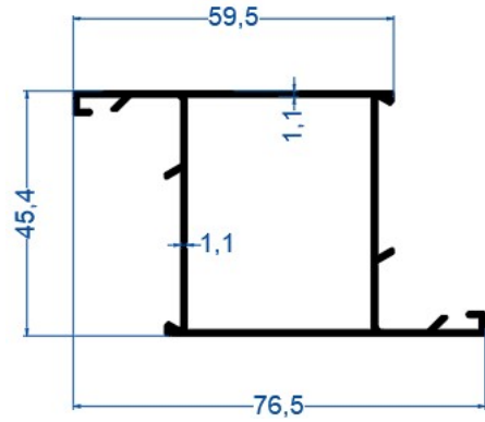
Aldoks Geniş Kanat Profili
