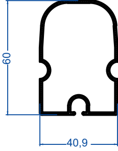
KÜÇÜK ARMUT PROFİLİ
