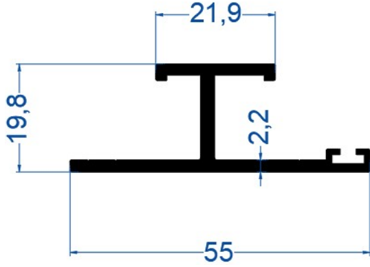
Sinter Klips Profil Tam
