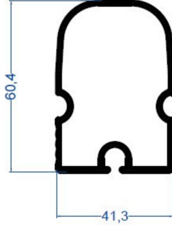
Küçük Armut Profili
