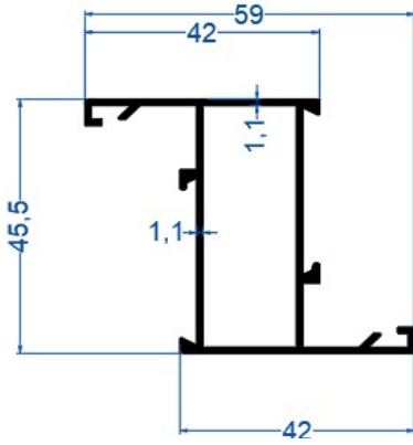
Aldoks Dar Kanat Profili
