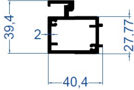
Hareketli Yan Kayıt Profili
