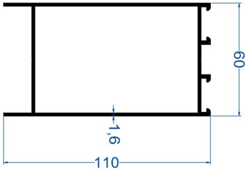
C-60 Etek Profili
