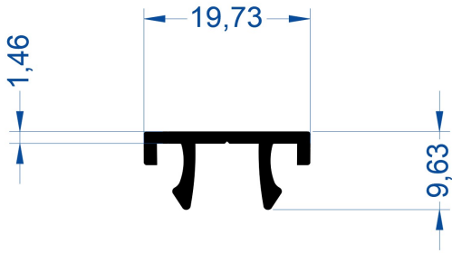
Pi Çıta Profili
