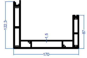
E-1016 5,170 kg/m Dere Profili
