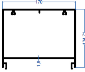
E-1012 3,810 kg/m Taşıyıcı Kutu Profili
