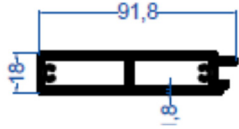
E-1015 1,268 kg/m Dere Ek & Taç Profili
